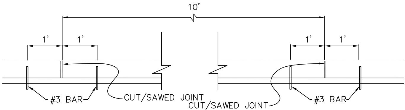
ELEVATION
