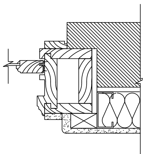
INTEGRAL TYPE JAMB
